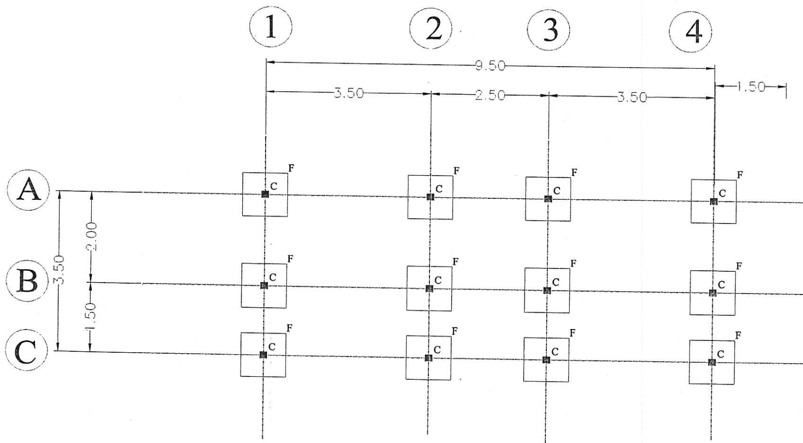
แปลนฐานราก และเสาตอม่อ นาคระส่วน 1:75
