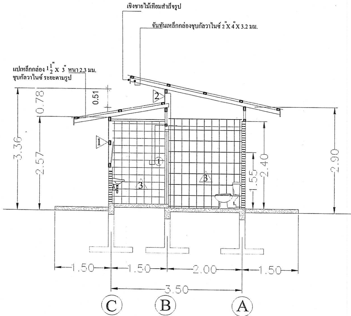
รูปตัด 1-1 มาตราส่วน 1:50
