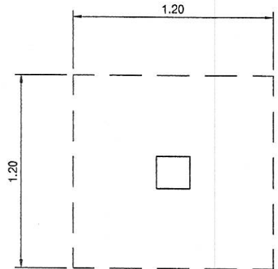
F1, C1 1:25
