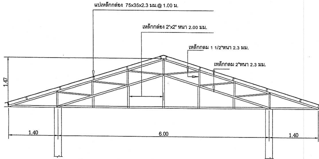
แบบขยาย T1
