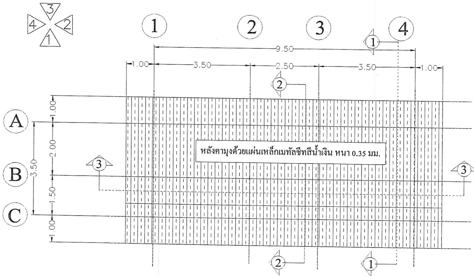
แปลนหลังคา มาตราส่วน 1:75
