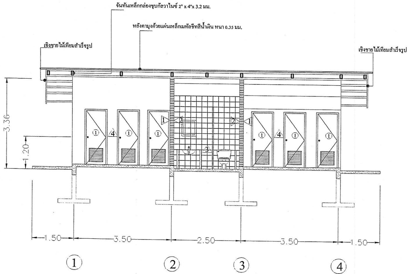
รูปตัด 3 - 3 มาตราส่วน 1:75
