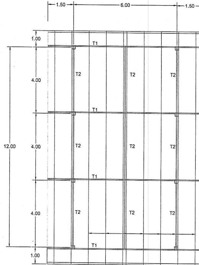
แปลนค้ำกึ่งตง 100 x 50 x 2.3 มม. @ 1.00 ม.
