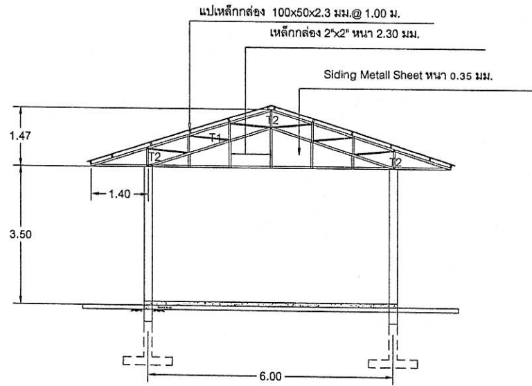
รูปตัด ก
