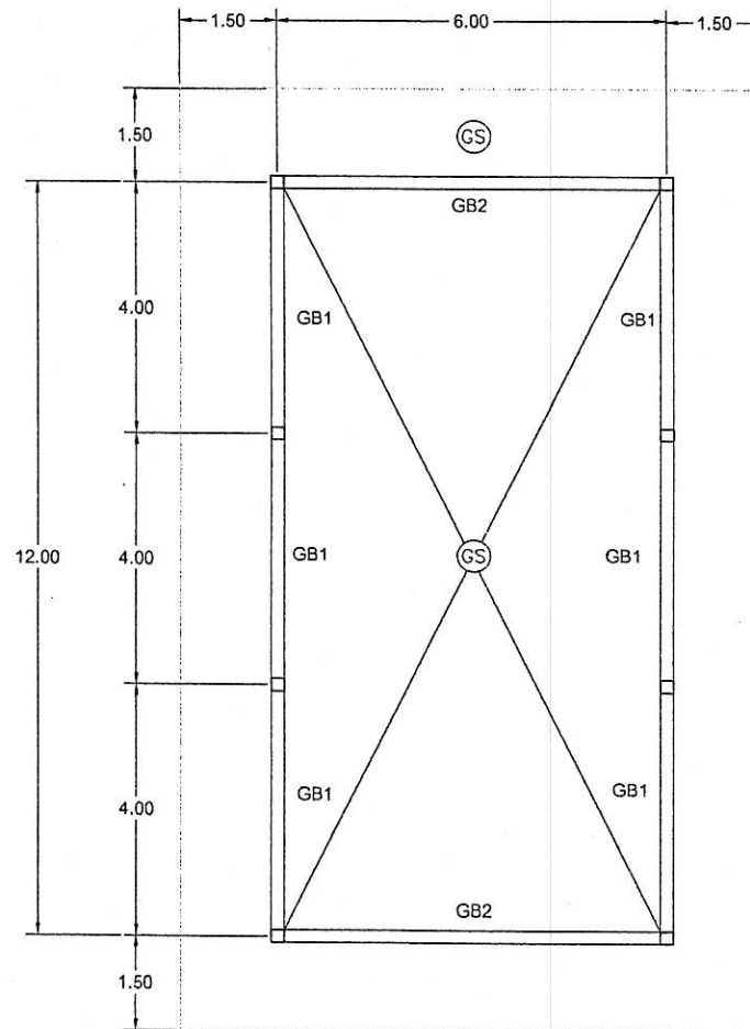
แปลนคานาคอดิน
