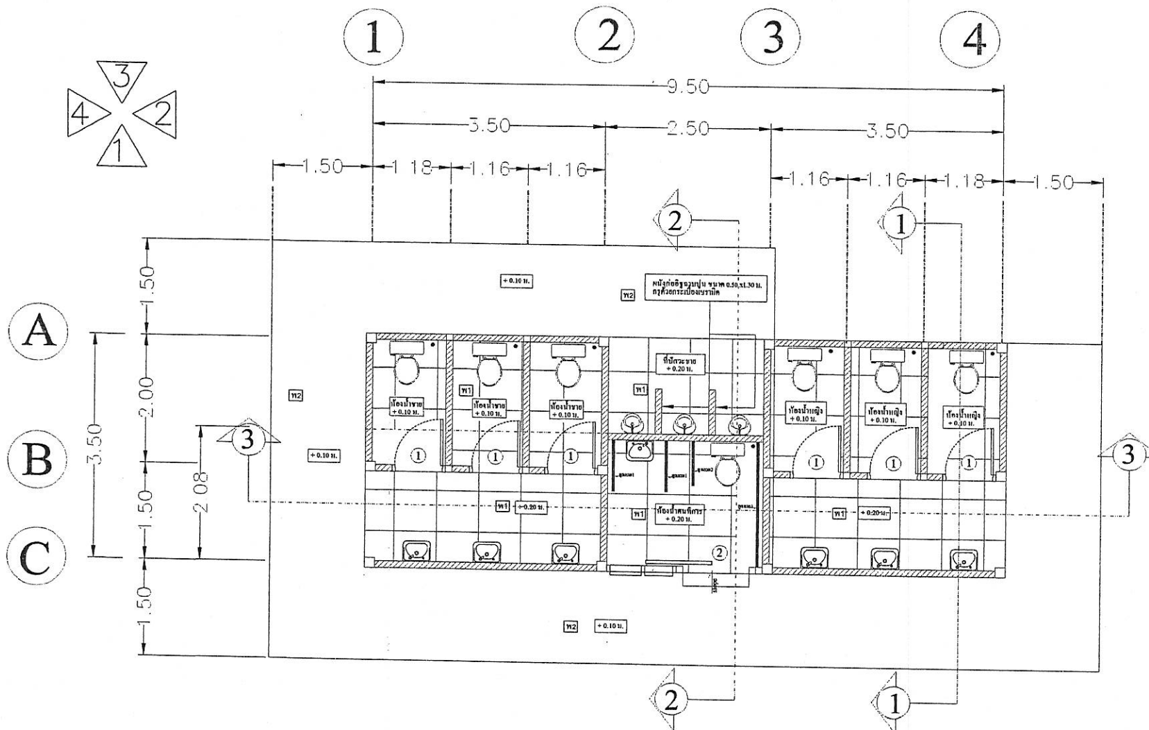
แปลนพื้นห้องน้ำ มาตราส่วน 1:75
