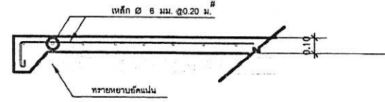
S1 1:25
