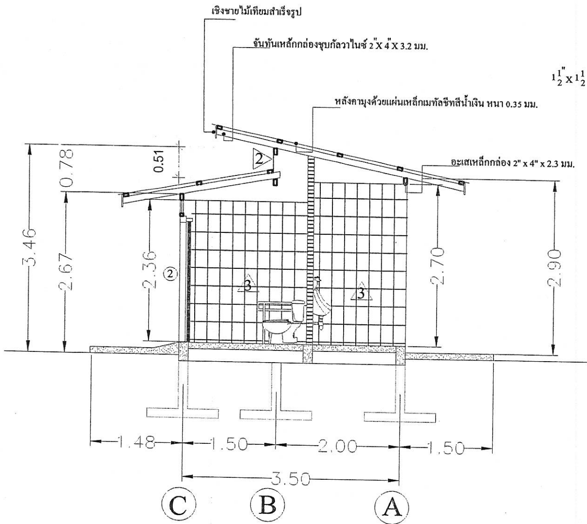
รูปตัด ② - ② มาตราส่วน 1:50
